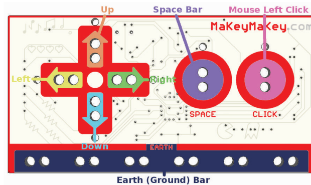
Gambar 9-2 Bagian Depan Papan Sirkuit Makey Makey
