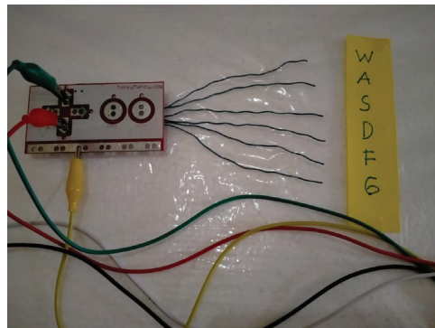
Gambar 9-6 Antarmuka dengan Makey Makey
