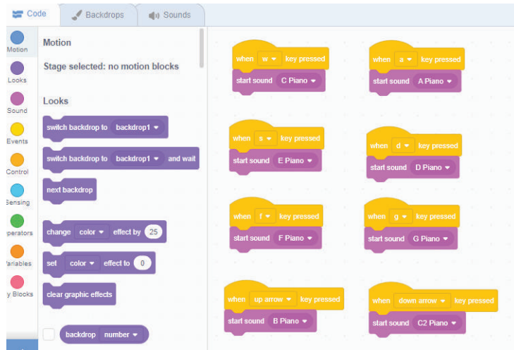
Gambar 9-5 Kode dengan Scratch Sumber: Dokumen Kemendikbud, 2021
